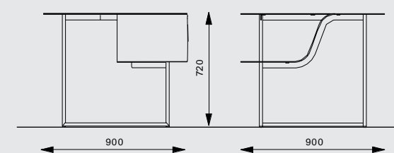
MNT190 MNT290
