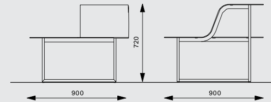
MNT170 MNT270
