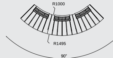
LVS32-e-t LVS32-e-twj
