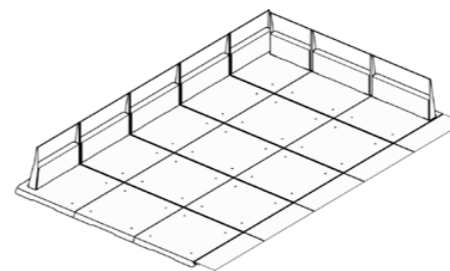
12 Moduli 7,20 x 4,68 m
