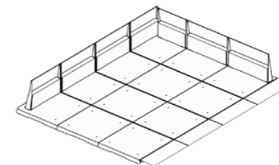
9 Moduli 5,76 x 4,68 m
