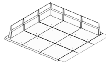
6 Moduli 4,32 x 4,68 m
